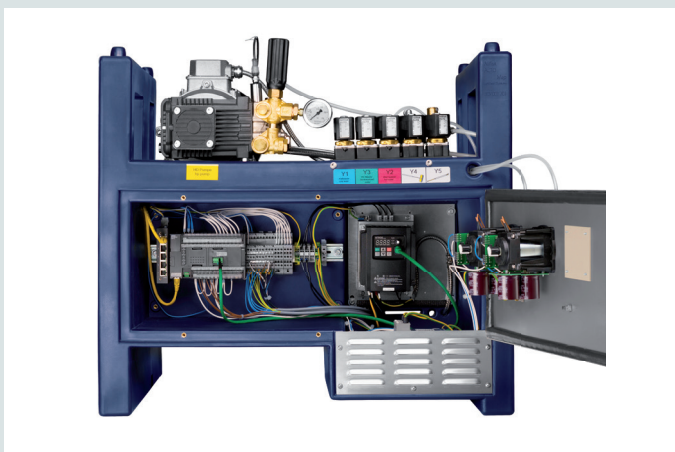
Pumpenmodul mit integrierter Steuerung
